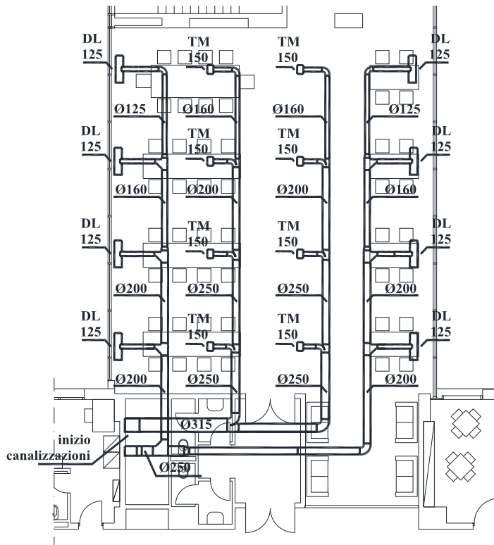
Figura 0.6 – Pianta con canalizzazioni dimensionate.
